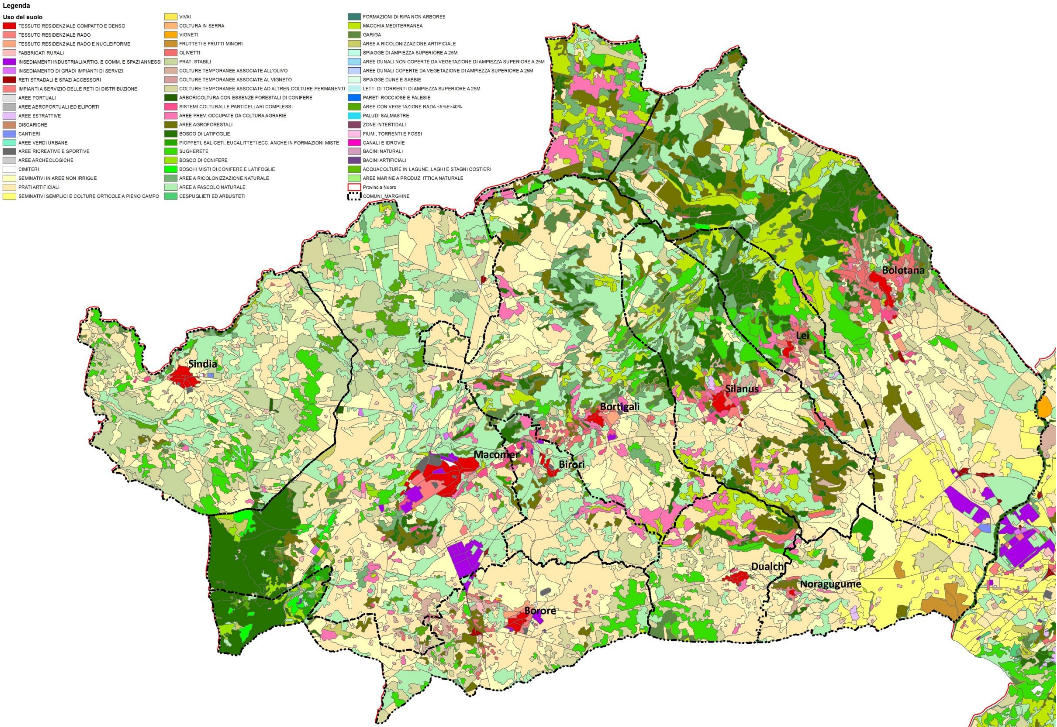
Figura 6. Uso del suolo.
